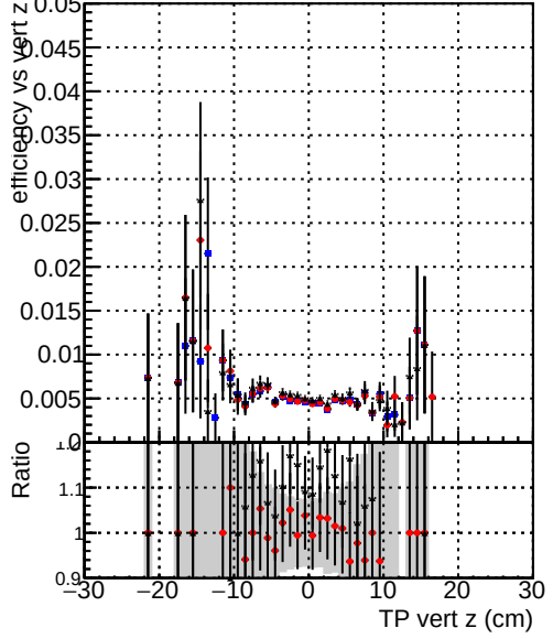
Efficiency vs. TP vert z (cm) Legend: - DQM_CKF_TTbase (blue circles) - DQM_CKF_TT_retrainOldFiles113 (red circles) - DQM_CKF_TT_retrainOldFiles125 (black circles)
