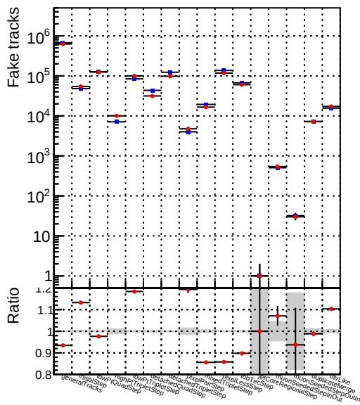
Number DOM mkFit XiMinusPU retrain 1 2 3 4 5 6 7 8 9 10 11 12 13 14 15 16 17 18 19 20 21 22 23 24 25 26 27 28 29 30 31 32 33 34 35 36 37 38 39 40 41 42 43 44 45 46 47 48 49 50 51 52 53 54 55 56 57 58 59 60 61 62 63 64 65 66 67 68 69 70 71 72 73 74 75 76 77 78 79 80 81 82 83 84 85 86 87 88 89 90 91 92 93 94 95 96 97 98 99 100
