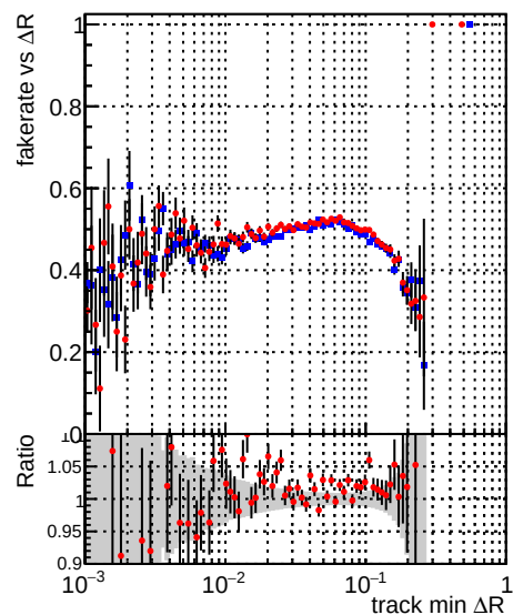
—•— DQM_mkFit_XiMinusPU_retrain —•— DQM_mkFit_XiMinusPU_retrain2
