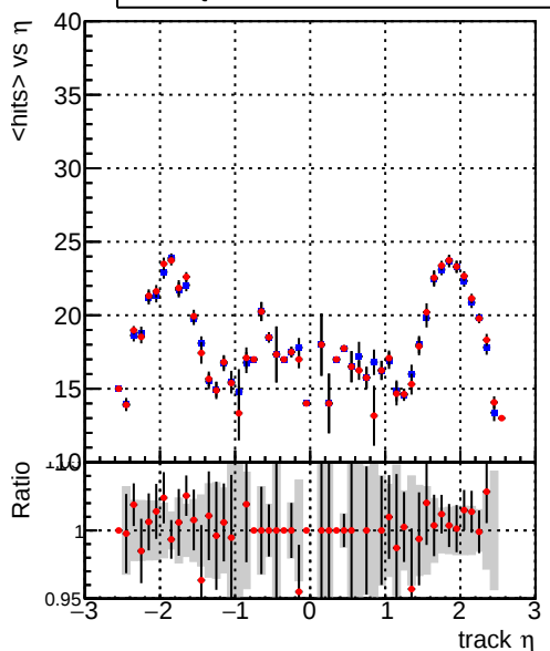
mean hit DQM_mkFit_XiMinusPU_retrain DQM_mkFit_XiMinusPU_retrain2
