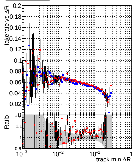
—■— DQM_mkFit_XiMinusPU_retrain —●— DQM_mkFit_XiMinusPU_retrain2
