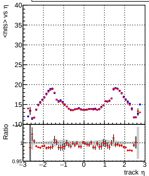
— DQM_mkFit_XiMinusPU_retrain — DQM_mkFit_XiMinusPU_retrain2 mean hits
