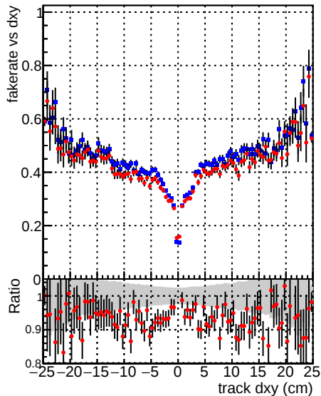
—◆— DQM_mkFit_XiMinusPU_retrain —◆— DQM_mkFit_XiMinusPU_retrain2
