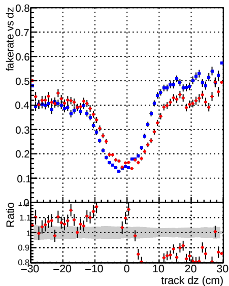
—◆— DQM_mkFit_XiMinusPU_retrain —◆— DQM_mkFit_XiMinusPU_retrain2
