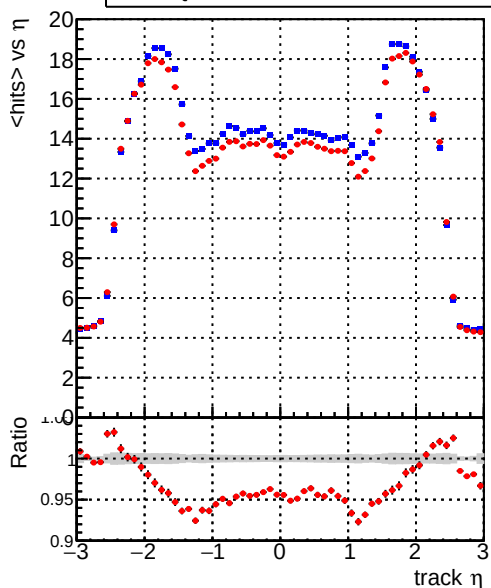
DQM_mkFit_XiMinusPU_retrain mean hits DQM_mkFit_XiMinusPU_retrain2
