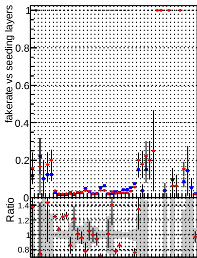
Fake rate vs. —■— DQM mkFit XiMinusPU_retrain —●— DQM mkFit XiMinusPU_retrain2
