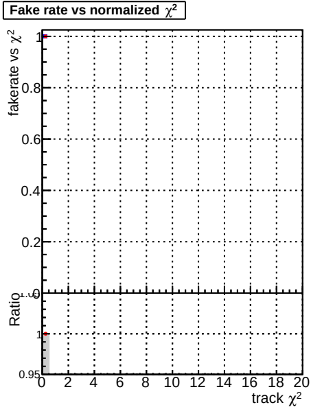
Fake rate vs. DQM_mkFit_XiMinusPU_retrain DQM_mkFit_XiMinusPU_retrain2
