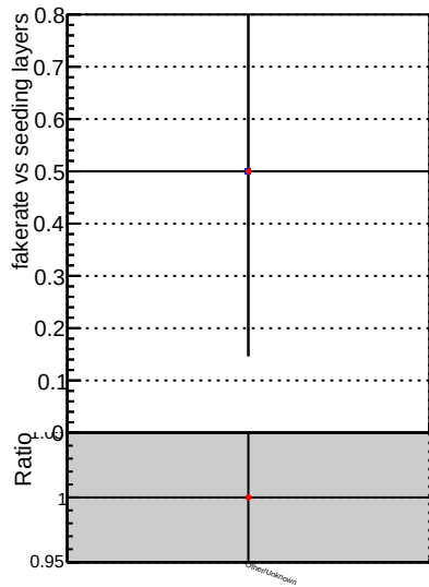
Fake rate vs. DQM_mkFit_XiMinusPU_retrain DQM_mkFit_XiMinusPU_retrain2
