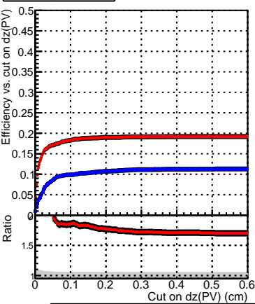
— DQM_mkFit_XiMinusPU_retrain — DQM_mkFit_XiMinusPU_retrain2
