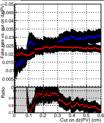
— DQM_mkFit_XiMinusPU_retrain — DQM_mkFit_XiMinusPU_retrain2
