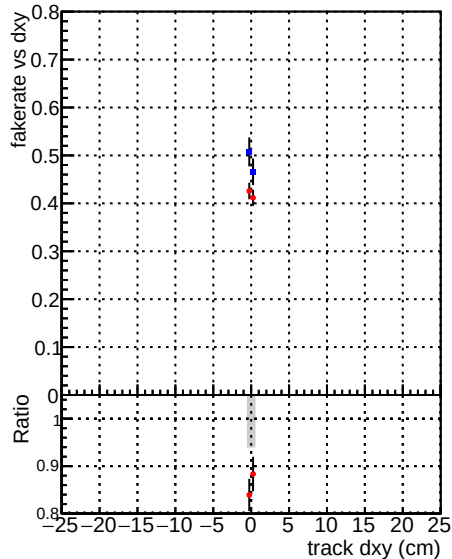
—●— DQM_mkFit_XiMinusPU_retrain —●— DQM_mkFit_XiMinusPU_retrain2
