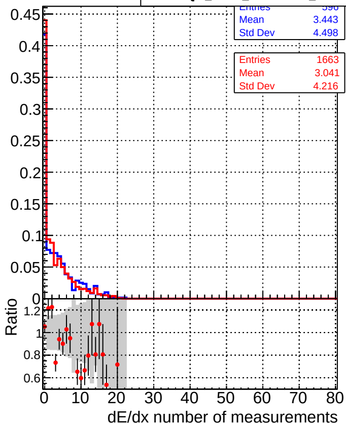
■ DQM_mkFit_XiMinusPU_retrain ● DQM_mkFit_XiMinusPU_retrain2
