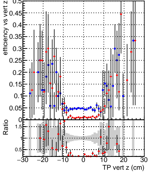
Efficiency vs vert z — DQM_mkFit_XiMinusPU_retrain — DQM_mkFit_XiMinusPU_retrain2
