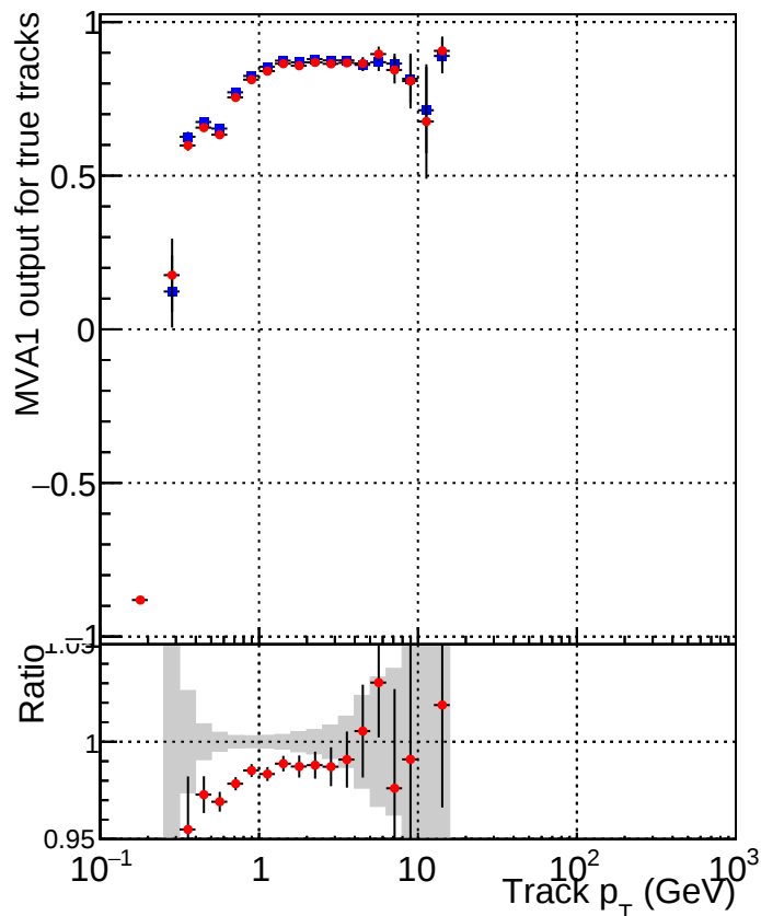
■ DQM_mkFit_XiMinusPU_retrain ■ DQM_mkFit_XiMinusPU_retrain2
