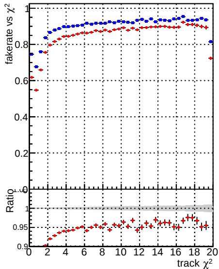
Fake rate vs. —•— DQM_mkFit_XiMinusPU_retrain —•— DQM_mkFit_XiMinusPU_retrain2
