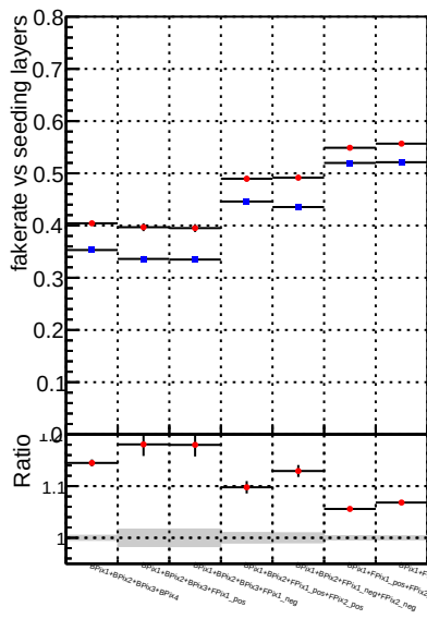
Fake rate vs. —●— DQM mkFit XiMinusPU_retrain —●— DQM mkFit XiMinusPU_retrain2
