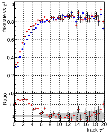
Fake rate vs. —●— DQM mkFit XiMinusPU_retrain —●— DQM mkFit XiMinusPU_retrain2
