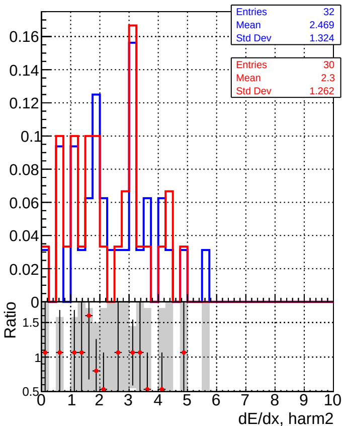
—■— DQM_mkFit_XiMinusPU_retrain —●— DQM_mkFit_XiMinusPU_retrain2
