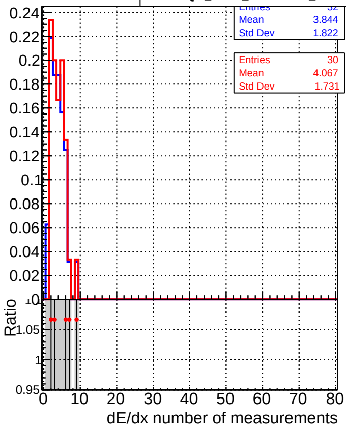
—■— DQM_mkFit_XiMinusPU_retrain —●— DQM_mkFit_XiMinusPU_retrain2
