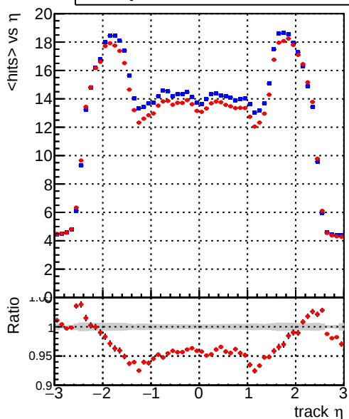
— DQM_mkFit_XiMinusPU_retrain — DQM_mkFit_XiMinusPU_retrain2 mean hits
