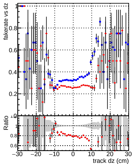
Fake rate vs dz —■— DQM mkFit XiMinusPU_retrain —●— DQM mkFit XiMinusPU_retrain2
