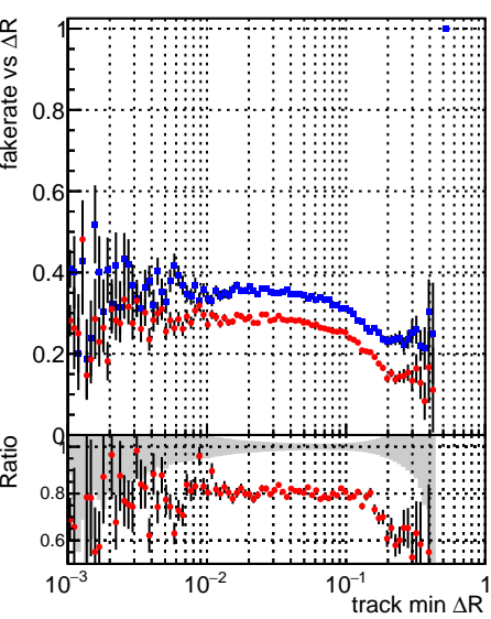
—•— DQM_mkFit_XiMinusPU_retrain —•— DQM_mkFit_XiMinusPU_retrain2
