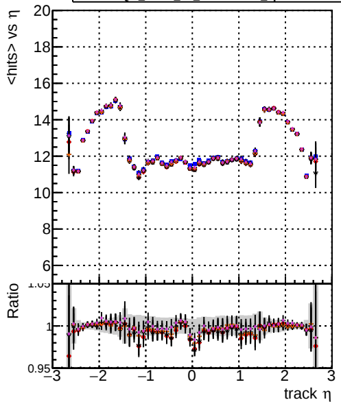
mean hits DQM mkFit TT NEWdefault specPless1-lowpt DQM mkFit TT NEWdefault specPless2-lowpt DQM mkFit TT NEWdefault specPless3-lowpt DQM mkFit TT NEWdefault specPless4-lowpt
