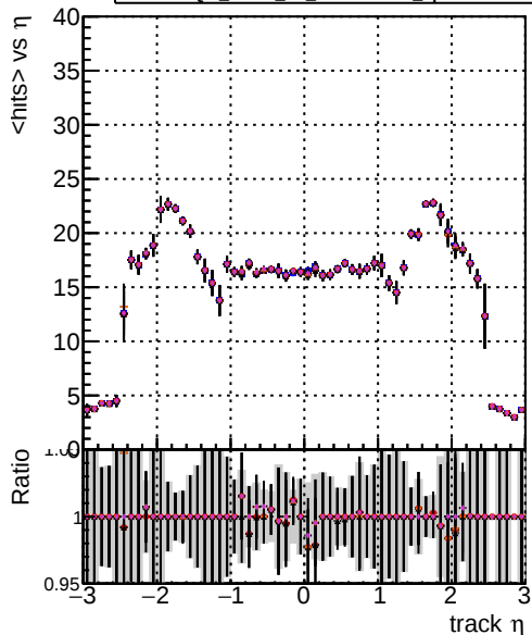
mean hits vs \eta DQM mkFit TT NEWdefault specPless1-lowpt DQM mkFit TT NEWdefault specPless2-lowpt DQM mkFit TT NEWdefault specPless3-lowpt DQM mkFit TT NEWdefault specPless4-lowpt
