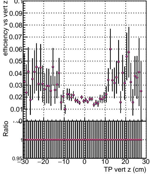
Efficiency vs vert z — DQM mkFit NEWdefault specPLess1-lowpt — DQM mkFit NEWdefault specPLess2-lowpt — DQM mkFit NEWdefault specPLess3-lowpt — DQM mkFit NEWdefault specPLess4-lowpt
