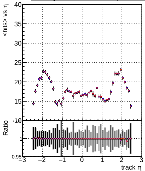
mean hits vs \eta DQM mkFit TT NEWdefault specPless1-lowpt DQM mkFit TT NEWdefault specPless2-lowpt DQM mkFit TT NEWdefault specPless3-lowpt DQM mkFit TT NEWdefault specPless4-lowpt
