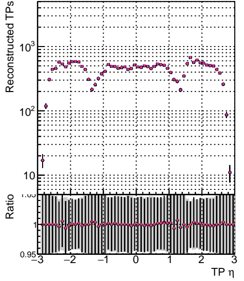
N of sim — DQM mkFit XiMinusPU NEWdefault specLess1 — DQM mkFit XiMinusPU NEWdefault specLess2 — DQM mkFit XiMinusPU NEWdefault specLess3 — DQM mkFit XiMinusPU NEWdefault specLess4
