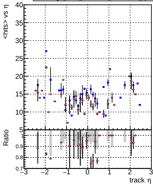
Legend: — DQM mkFit XiMinusPU NEWdefault specPless1 — DQM mkFit XiMinusPU NEWdefault specPless2 — DQM mkFit XiMinusPU NEWdefault specPless3 — DQM mkFit XiMinusPU NEWdefault specPless4
