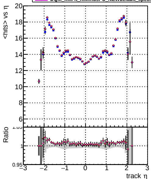
mean hits DQM mkFit XiMinusPU NEWdefault specPLess1 DQM mkFit XiMinusPU NEWdefault specPLess2 DQM mkFit XiMinusPU NEWdefault specPLess3 DQM mkFit XiMinusPU NEWdefault specPLess4
