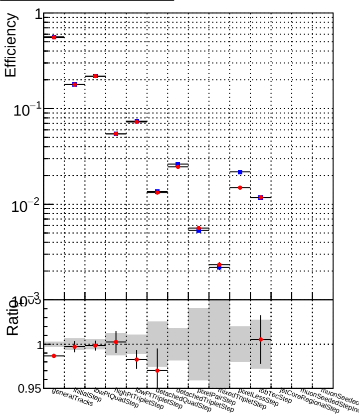
DQM_mkFit_XiMinusPU_retrain2 DQM_mkFit_XiMinusPUold
