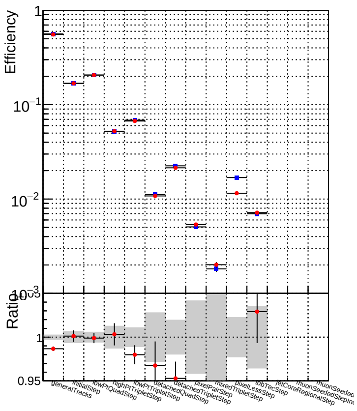
DQM_mkFit_XiMinusPU_retrain2 DQM_mkFit_XiMinusPUold
