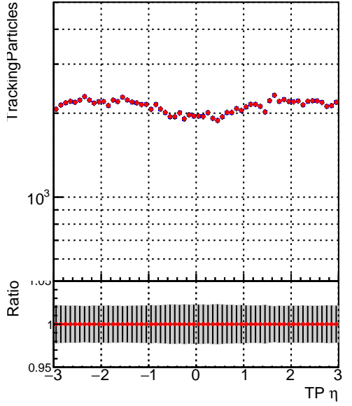
■ DQM_mkFit_XiMinusPU_retrain2 ■ DQM_mkFit_XiMinusPUold
