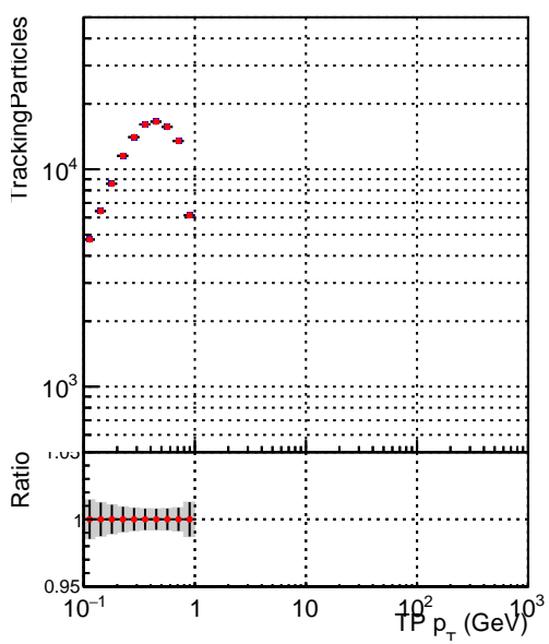
■ DQM_mkFit_XiMinusPU_retrain2 ● DQM_mkFit_XiMinusPUold
