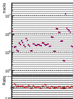
N of reco track vs. \chi^2 —•— DQM_mkFit_XiMinusPU_retrain2 —•— DQM_mkFit_XiMinusPUold
