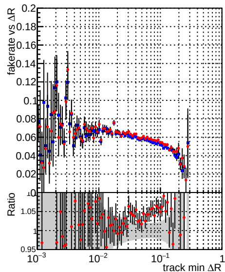
—●— DQM_mkFit_XiMinusPU_retrain2 —●— DQM_mkFit_XiMinusPUold
