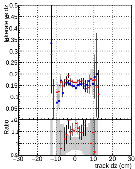
—●— DQM_mkFit_XiMinusPU_retrain2 —●— DQM_mkFit_XiMinusPUold
