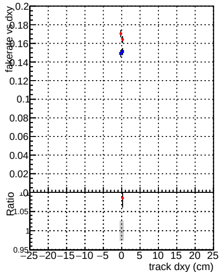
—●— DQM_mkFit_XiMinusPU_retrain2 —●— DQM_mkFit_XiMinusPUold
