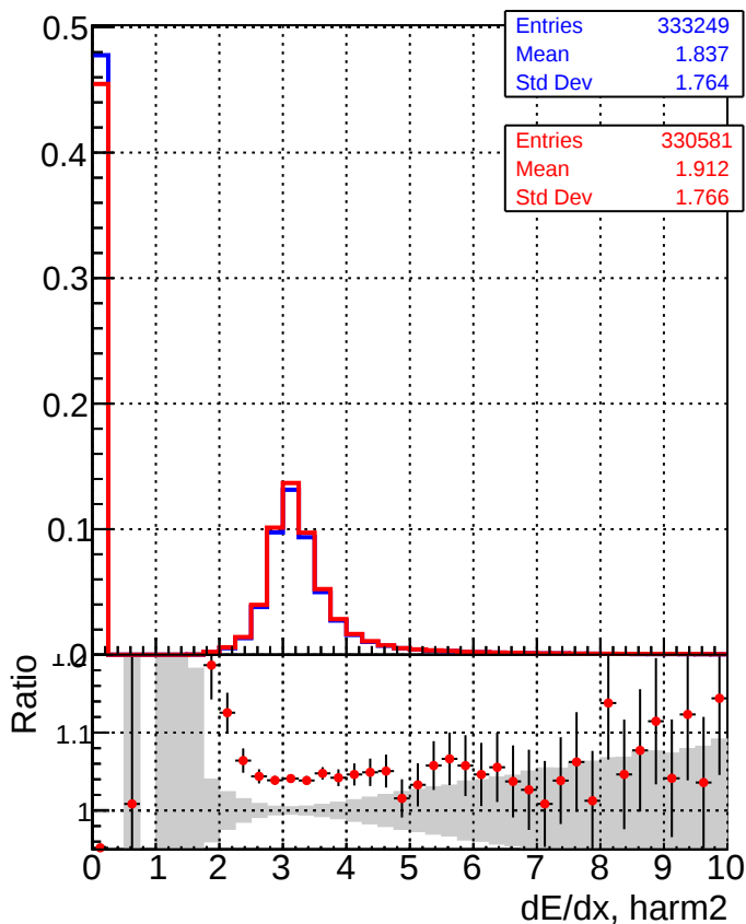
DQM_mkFit_XiMinusPU_retrain2 DQM_mkFit_XiMinusPUold
