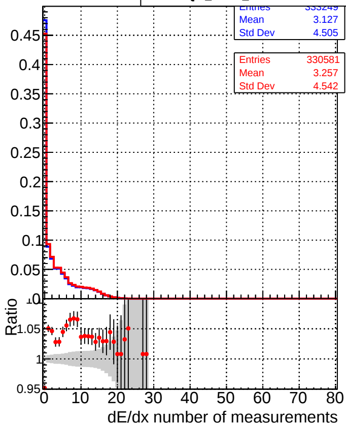
DQM_mkFit_XiMinusPU_retrain2 DQM_mkFit_XiMinusPUold
