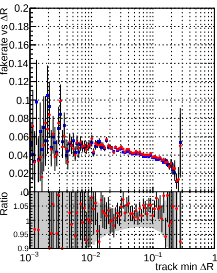
Legend: \blacksquare DQM_mkFit_XiMinusPU_retrain2 \bullet DQM_mkFit_XiMinusPUold
