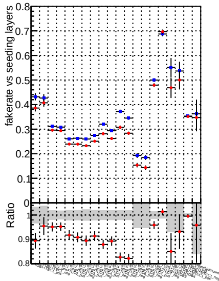
Fake rate vs. —◆— DQM_mkFit_XiMinusPU_retrain2 —●— DQM_mkFit_XiMinusPUold
