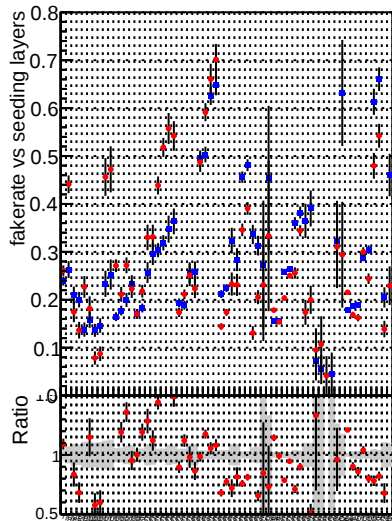
Fake rate vs. —◆— DQM_mkFit_XiMinusPU_retrain2 —★— DQM_mkFit_XiMinusPUold
