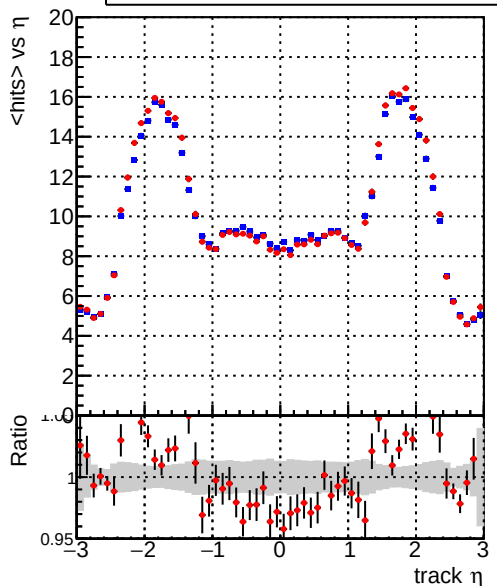
mean hit — DQM_mkFit_XiMinusPU_retrain2 — DQM_mkFit_XiMinusPUold
