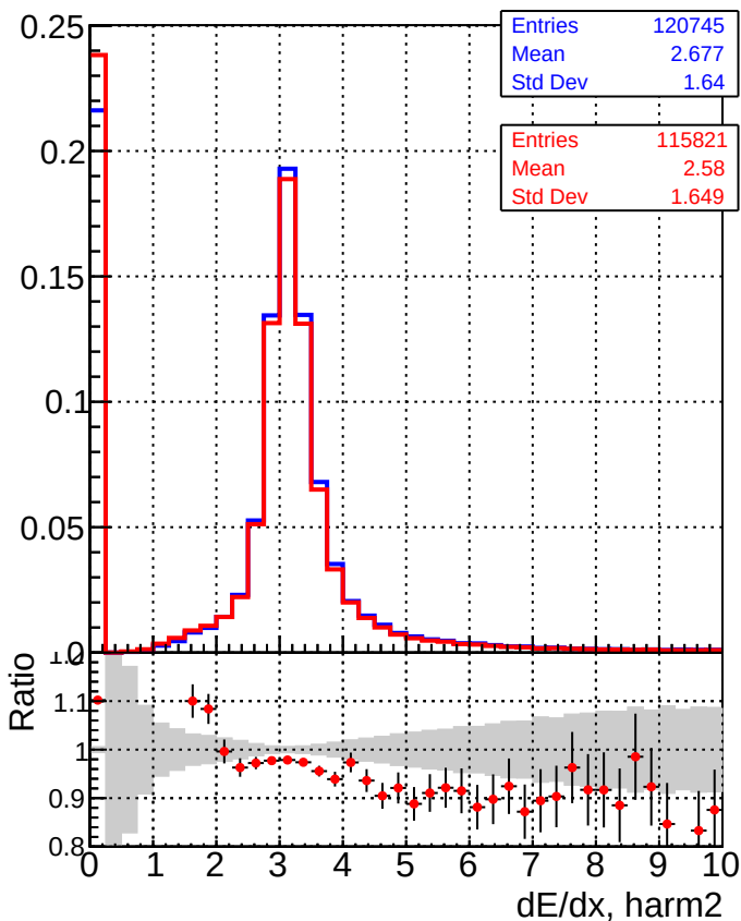
DQM_mkFit_XiMinusPU_retrain2 DQM_mkFit_XiMinusPUold
