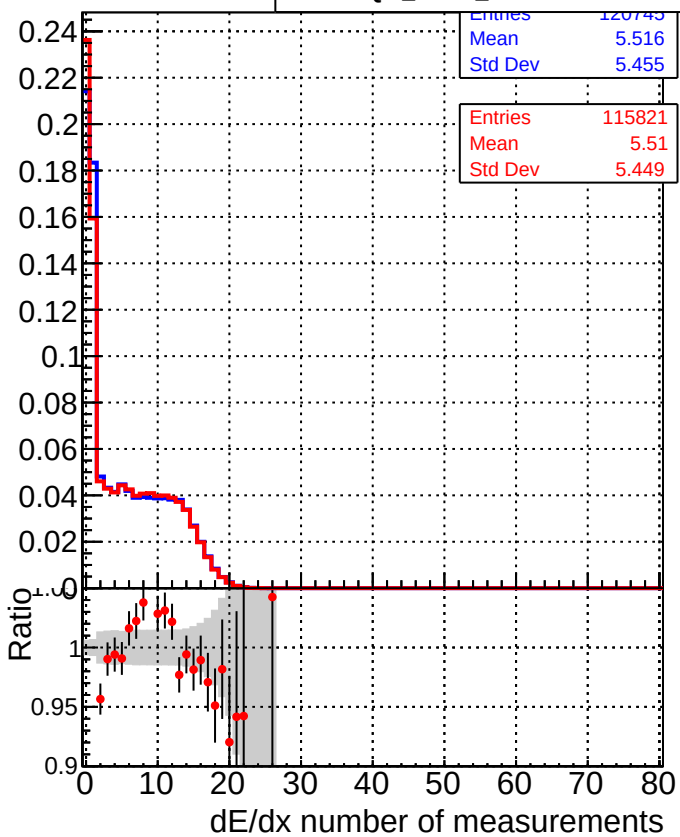
DQM_mkFit_XiMinusPU_retrain2 DQM_mkFit_XiMinusPUold
