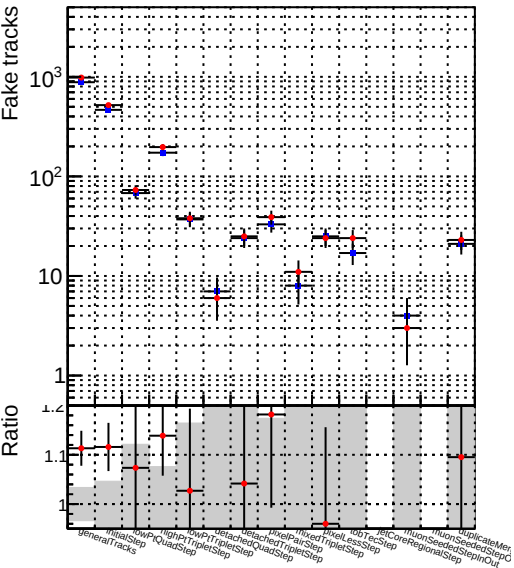
Number —●— DQM_mkFit_XiMinusPUold
