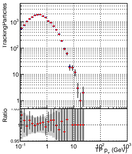
—•— DQM_mkFit_XiMinusPU_retrain2 —•— DQM_mkFit_XiMinusPUold
