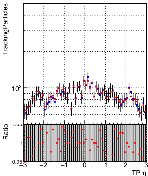
—•— DQM_mkFit_XiMinusPU_retrain2 —•— DQM_mkFit_XiMinusPUold
