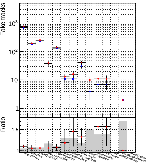
Number —●— DQM_mkFit_XiMinusPUold
