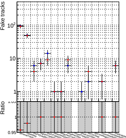
Number —●— DQM_mkFit_XiMinusP
