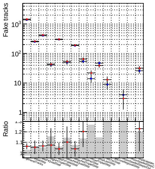
Number —●— DQM_mkFit_XiMinusPUold
