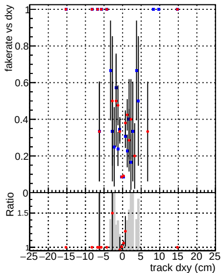
—●— DQM_mkFit_XiMinusPU_retrain2 —●— DQM_mkFit_XiMinusPUold
