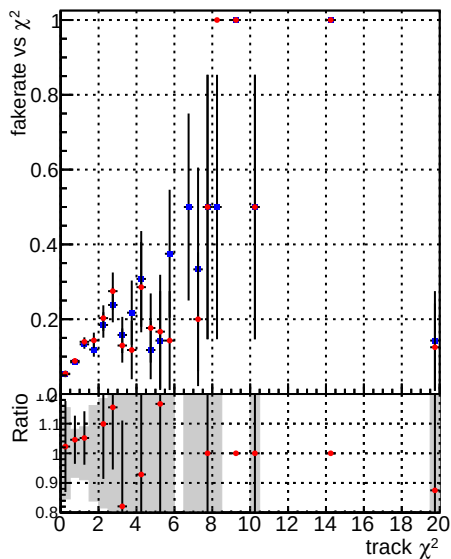
Fake rate vs. \chi^2 —•— DQM_mkFit_XiMinusPU_retrain2 —•— DQM_mkFit_XiMinusPUold
