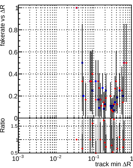
Fake rate vs ΔR(track, jet) DQM_mkFit_XiMinusPU_retrain2 DQM_mkFit_XiMinusPUold
