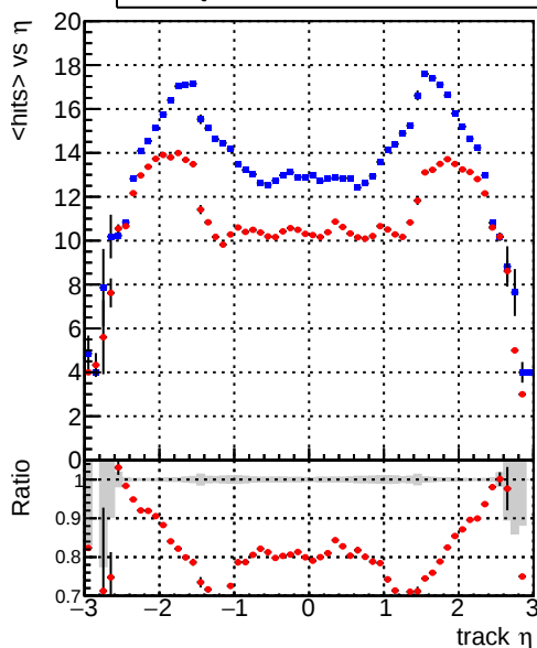
DQM_mkFit_XiMinusPU_retrain2 mean hit DQM_mkFit_XiMinusPUold
